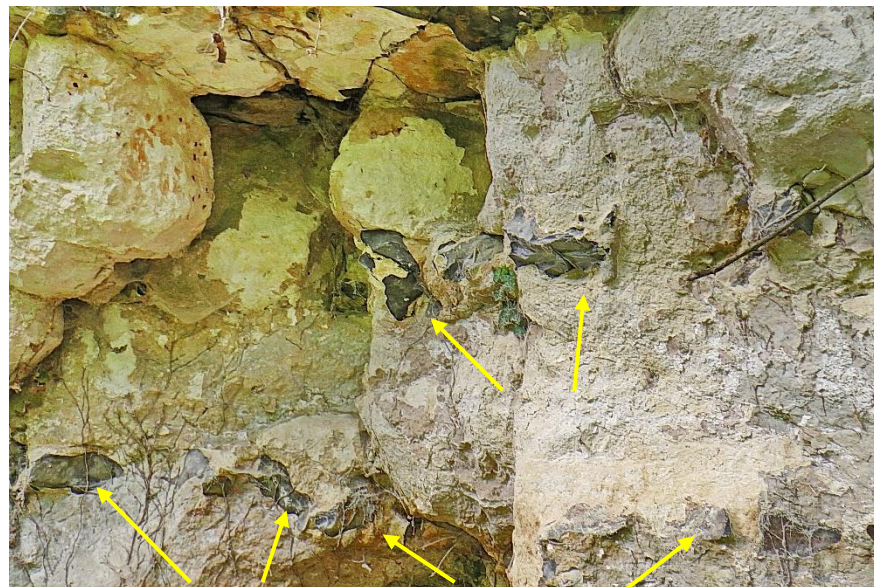
Nodules de silex dans la craie
